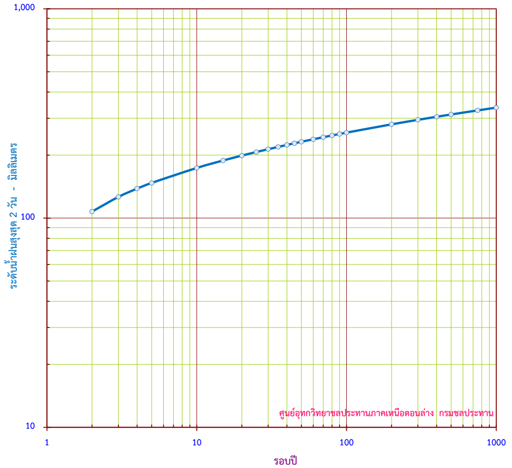
กราฟแสดง ปริมาณน้ำฝนสูงสุด 2 วัน ขนาดรอบปีต่างๆ สถานี 700221 อ.ตรอน จ.อุดรดิตถ์
